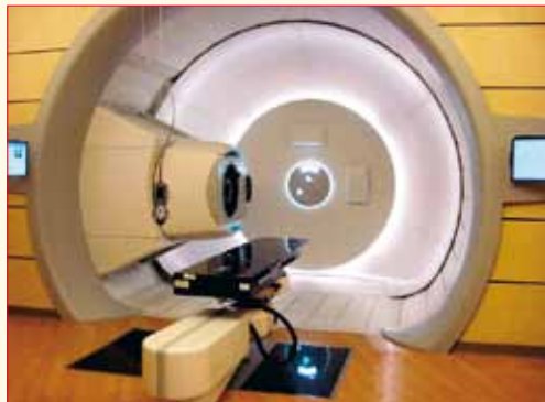
Les portiques rotatifs ou gantry room .
